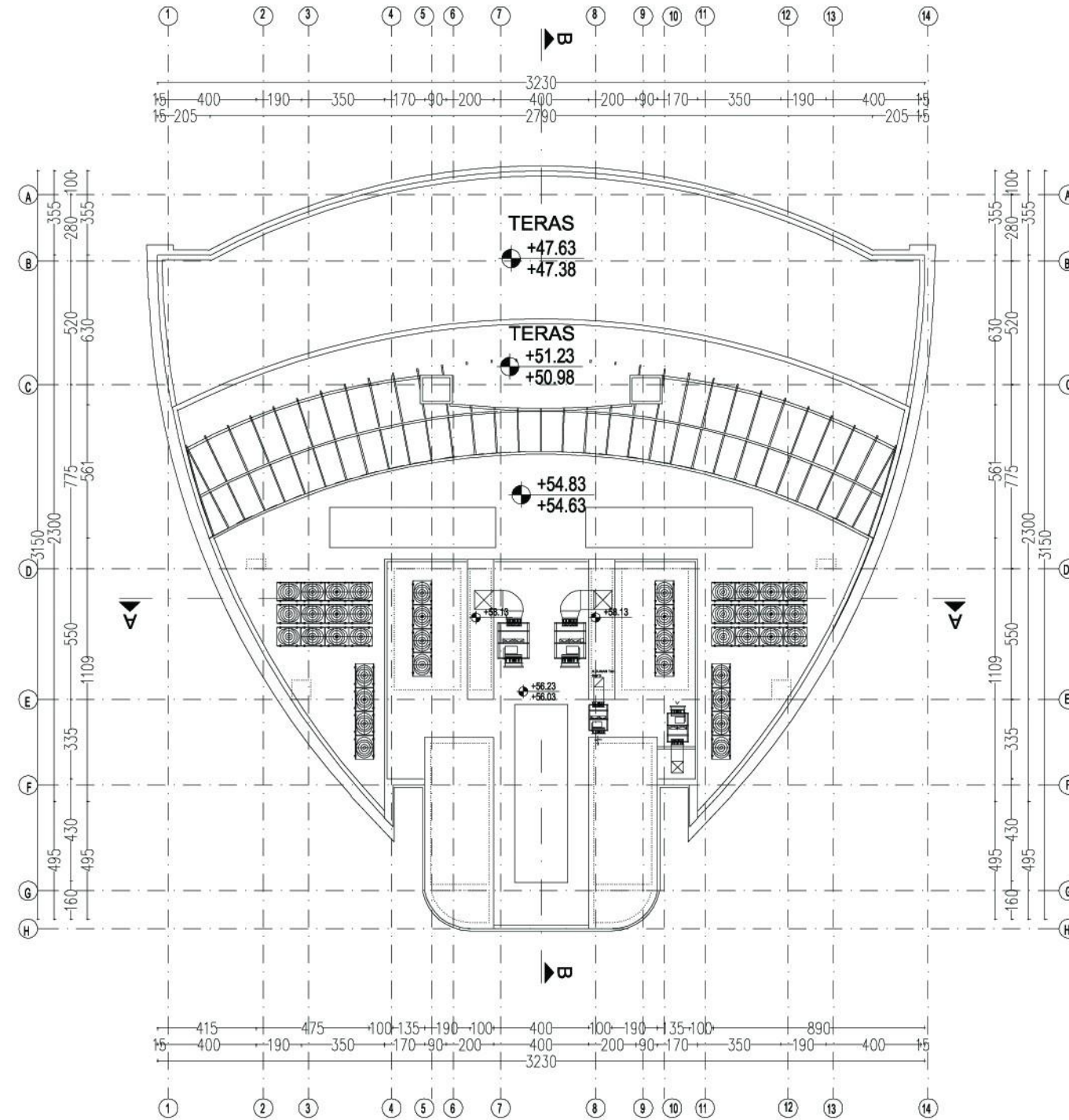
ÇATI KATI
