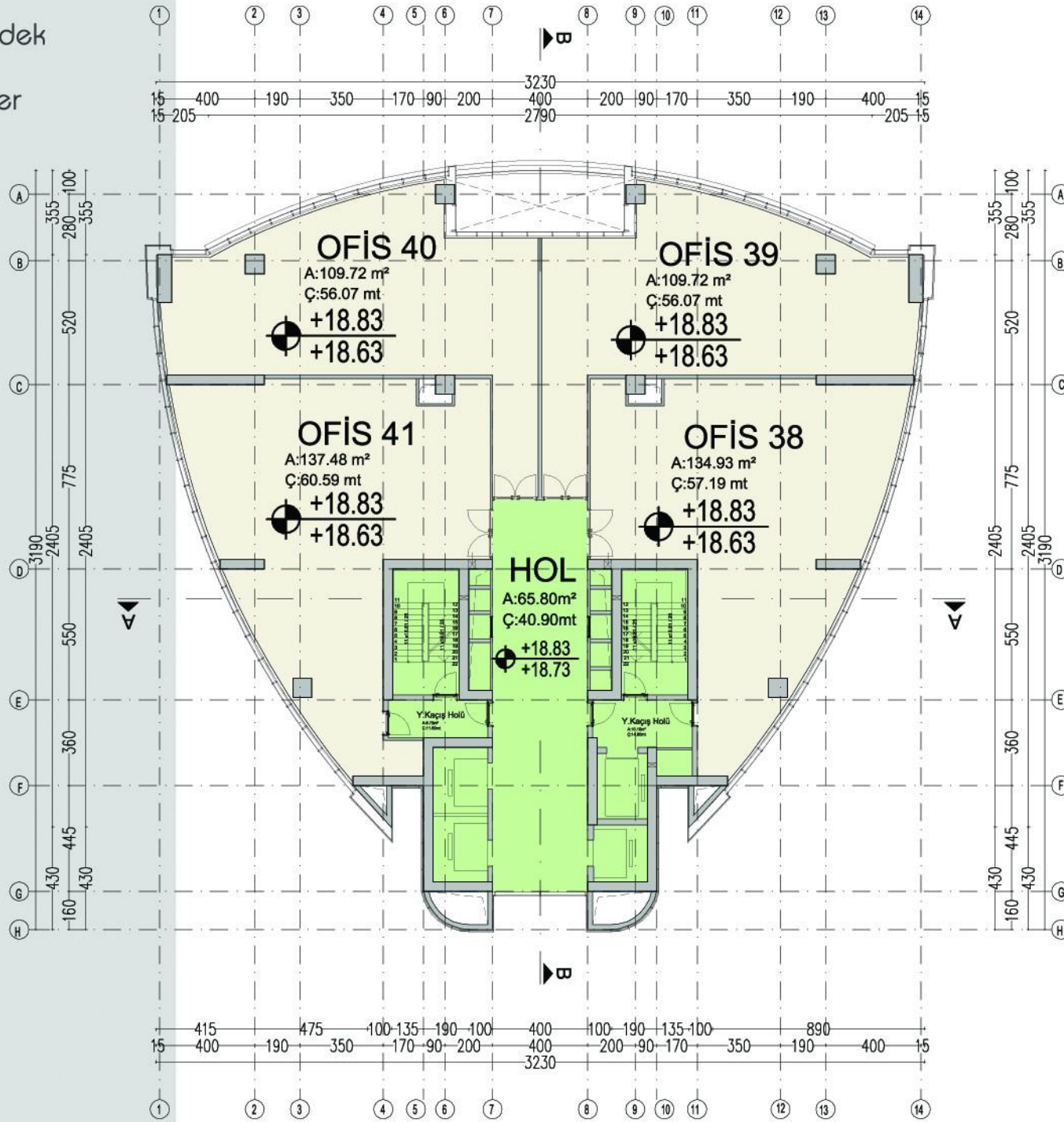
5.NORMAL KAT
