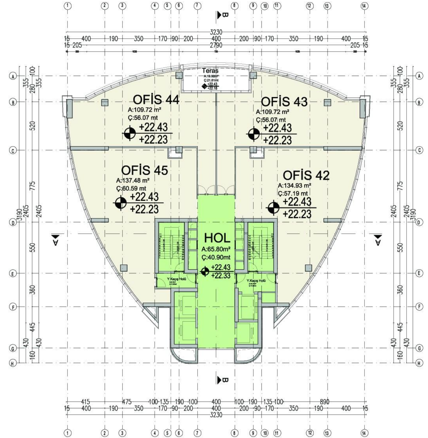
6.NORMAL KAT
