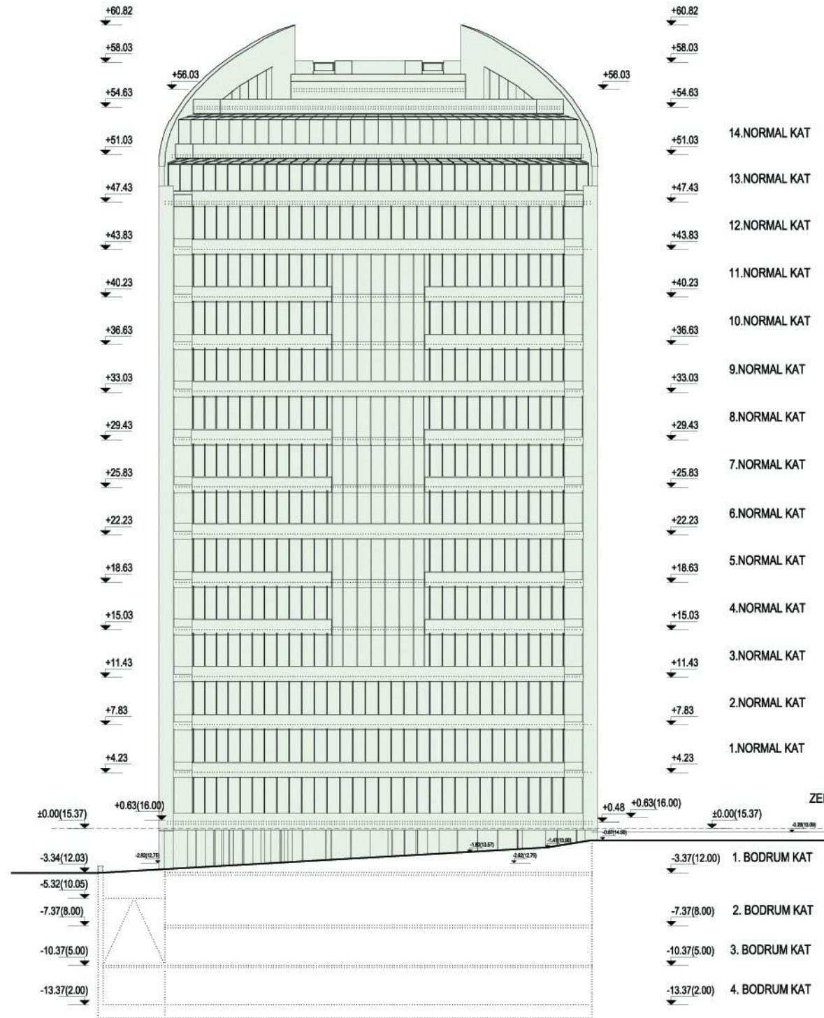
ÖN CEPHE
