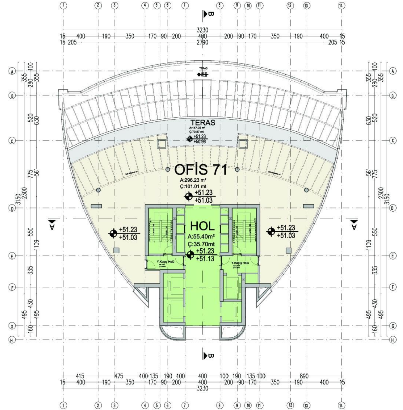
14.NORMAL KAT
