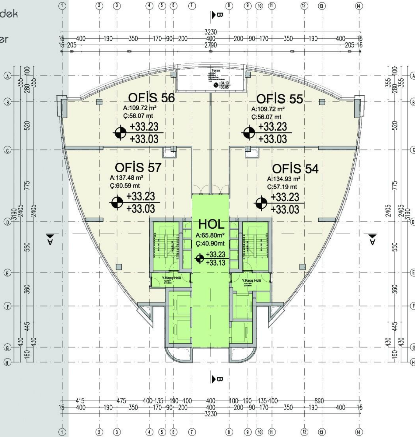
9.NORMAL KAT
