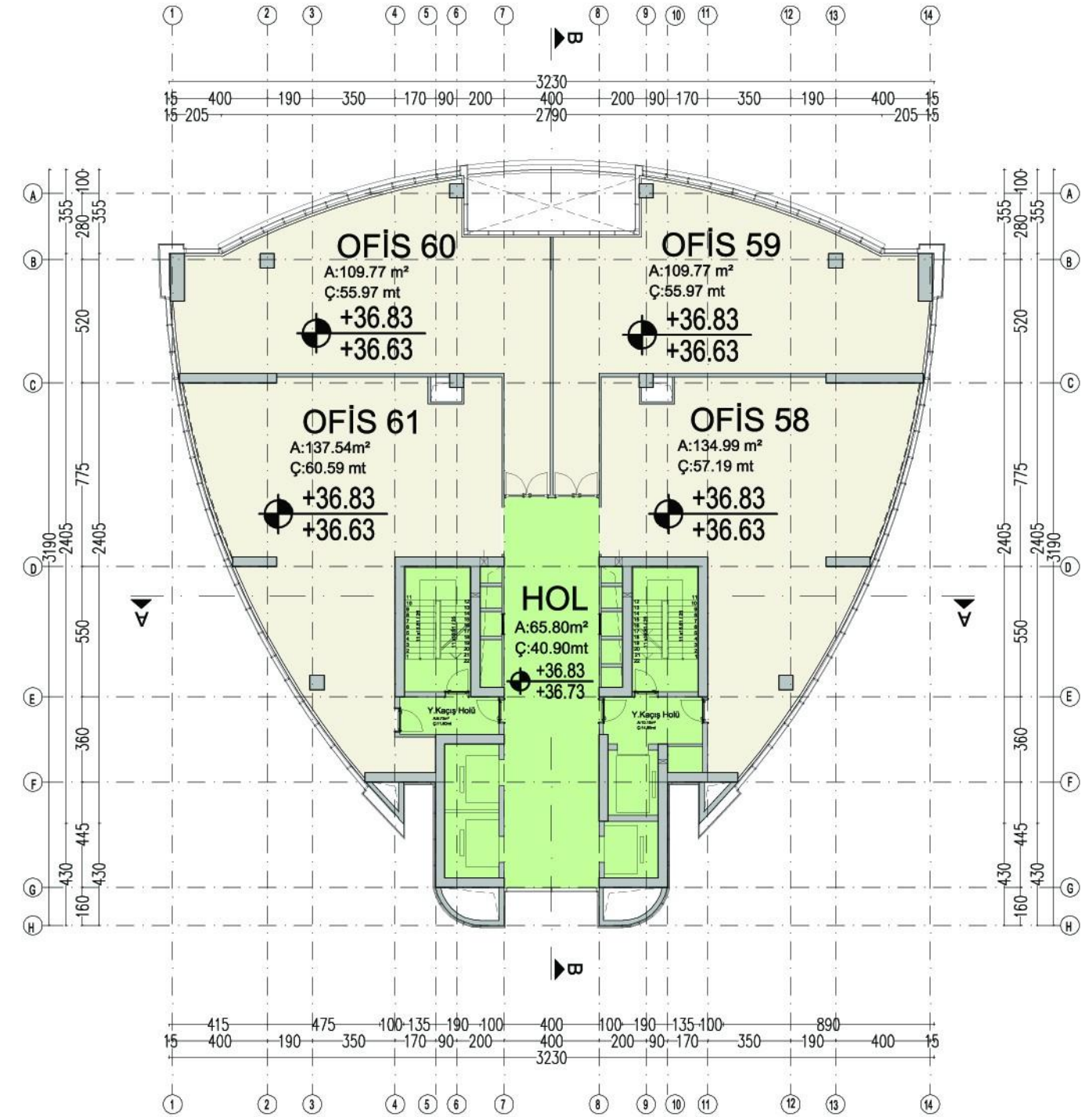
10.NORMAL KAT
