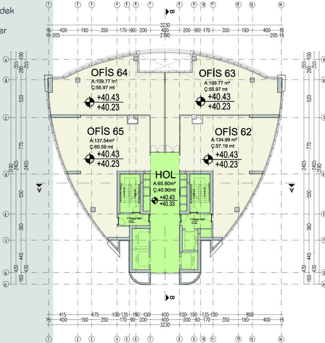
11. NORMAL KAT
