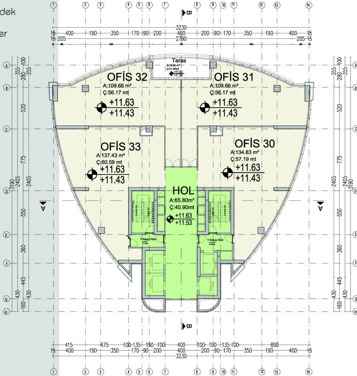
3.NORMAL KAT
